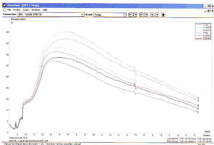
Rys. 5. Wyniki monitoringu przebiegu temperatury wewnątrz słupów głównych ramy o przekroju 0,80x1,80 m, przeprowadzonego w dniu 18 stycznia 2007 r.
